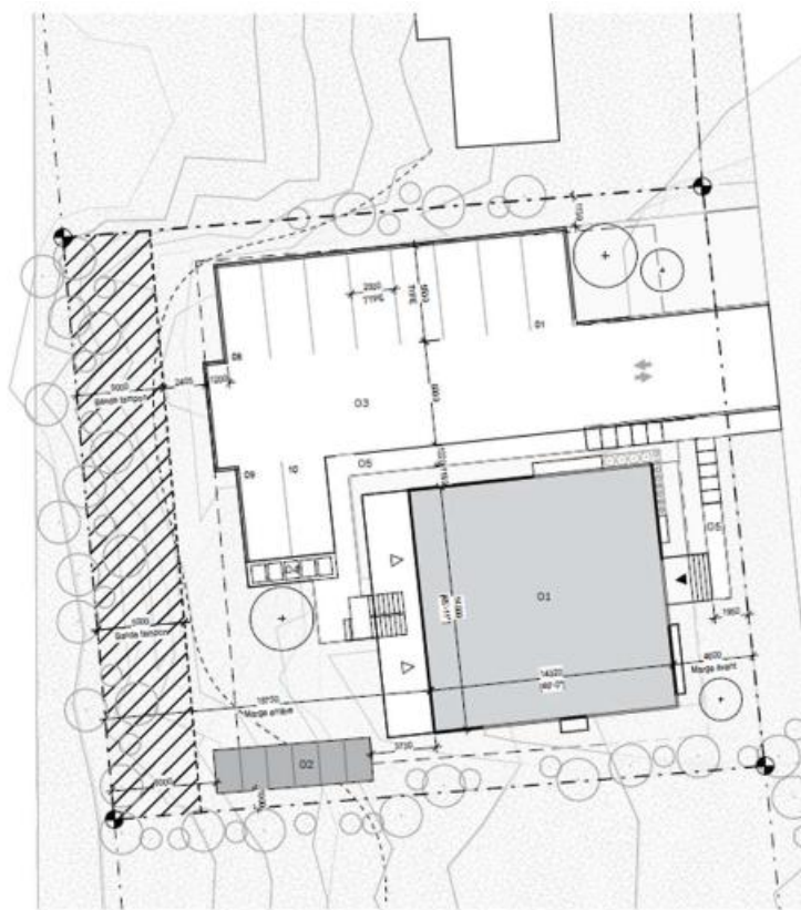
Plan d'implantation
